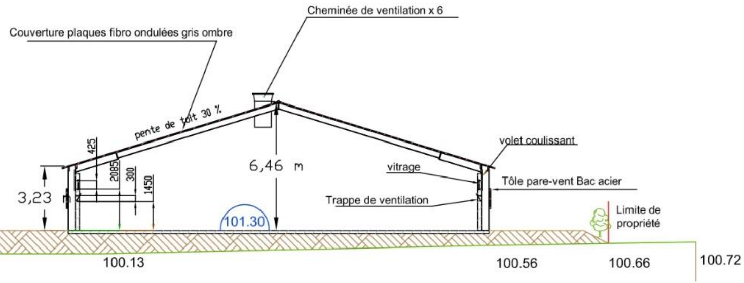
COUPE AB
